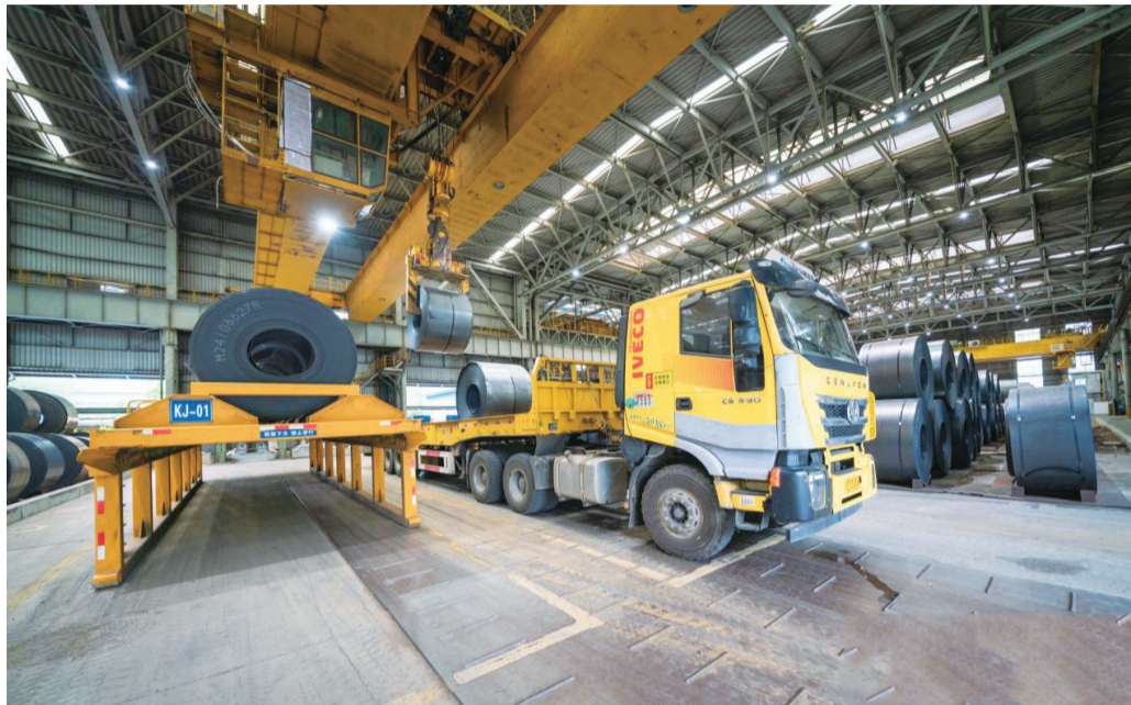
7月13日,位于马鞍山的宝武马钢四钢轧总厂1580生产线正在发运热轧板卷。入夏以来,工人们坚守岗位,聚焦“高品质、高效率、低消耗”,围绕品种结构、介质能源消耗等重点指标持续发力,奋力推动高质量发展。 张明伟 摄
